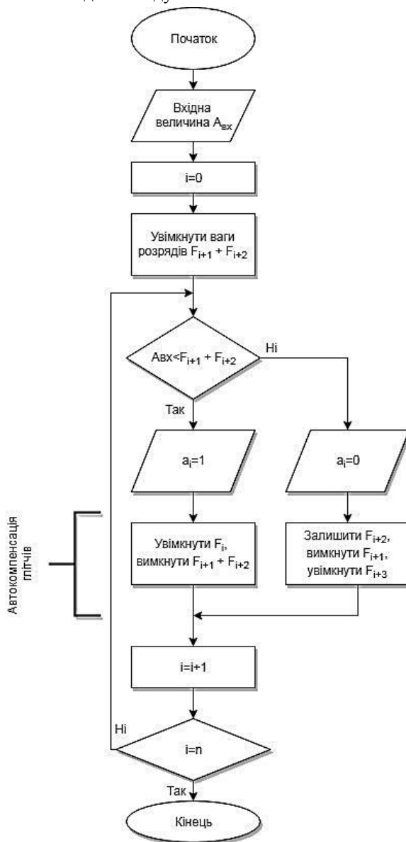
Рисунок 2. Модифікований алгоритм послідовного наближення в АЦП з НПСЧ з автокомпенсацією глітчів
